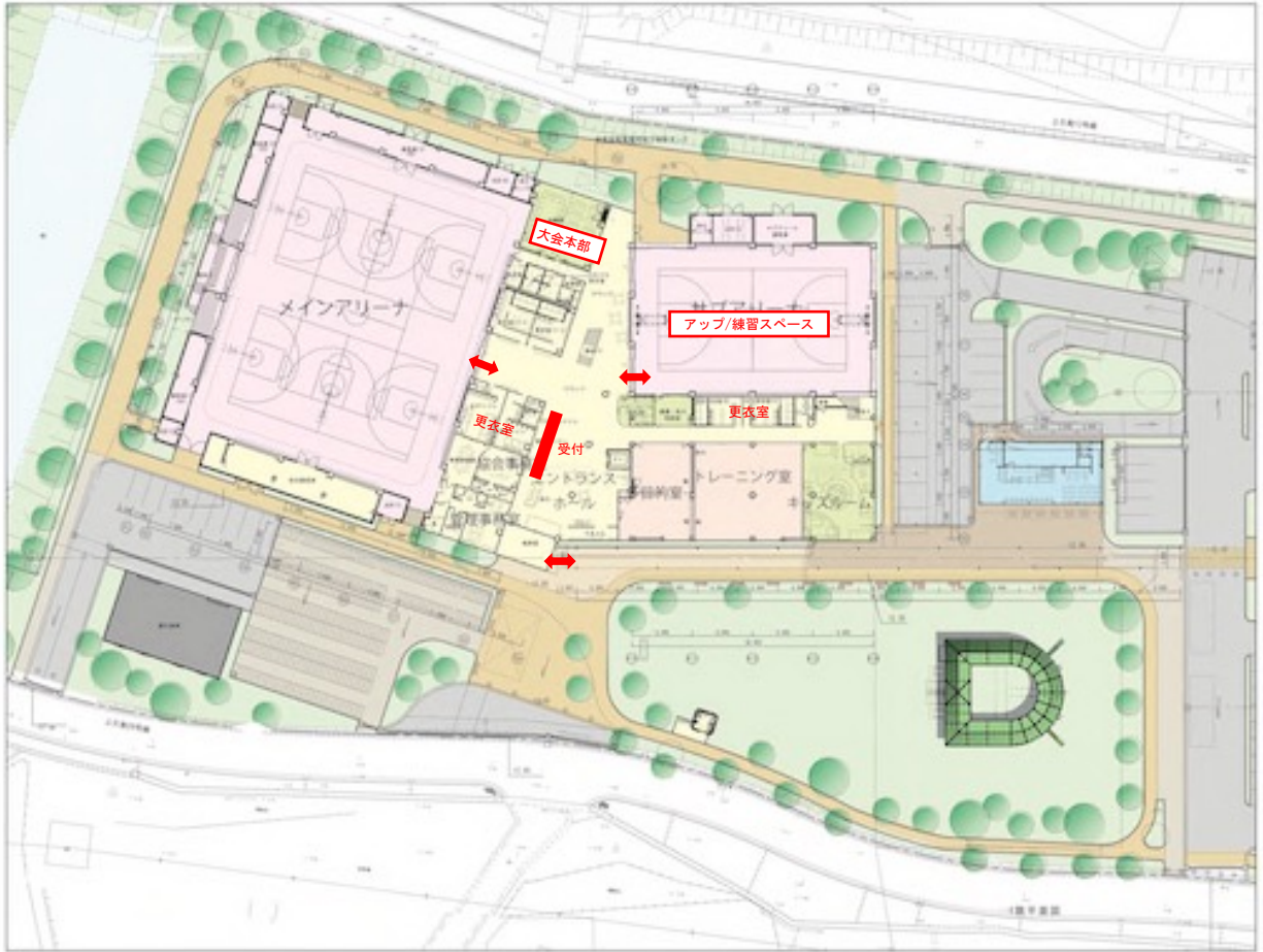
【1F平面図】
