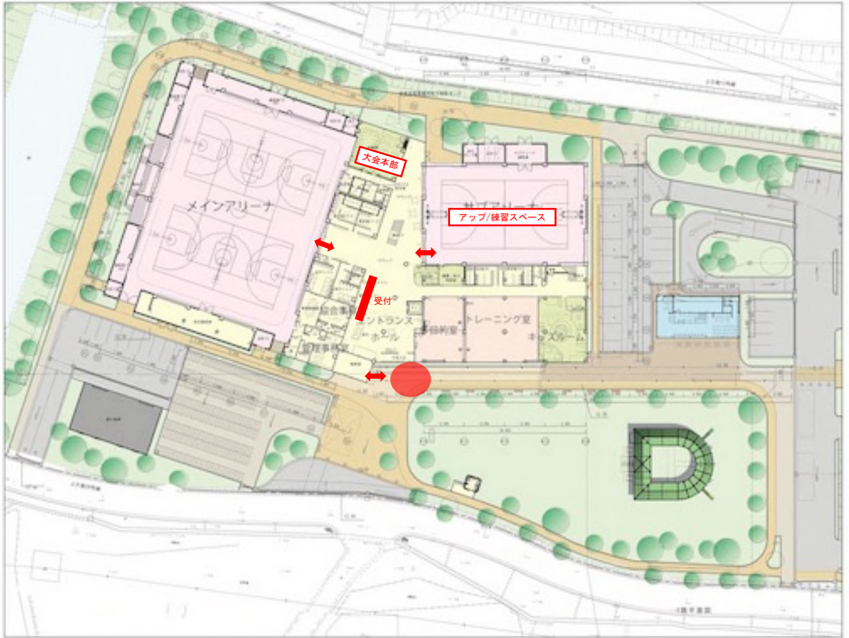
【1F平面図】
