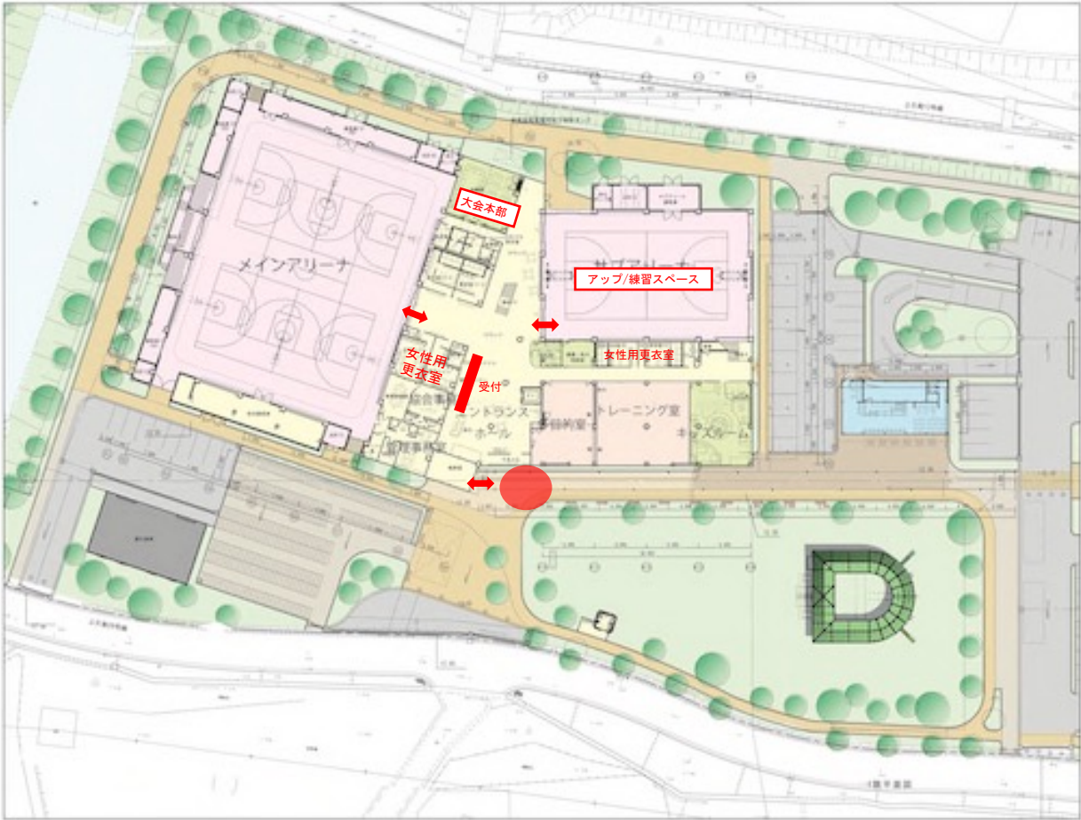
【1F平面図】
